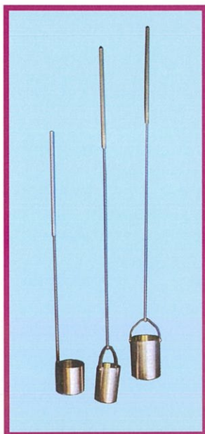
左:ディッパー<全体図> 上:可動式ディッパー <可動時>
